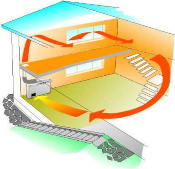
TVÅVÅNINGSPÅN/SOUTERÅNG Installation med kort kanal i nedre plan
