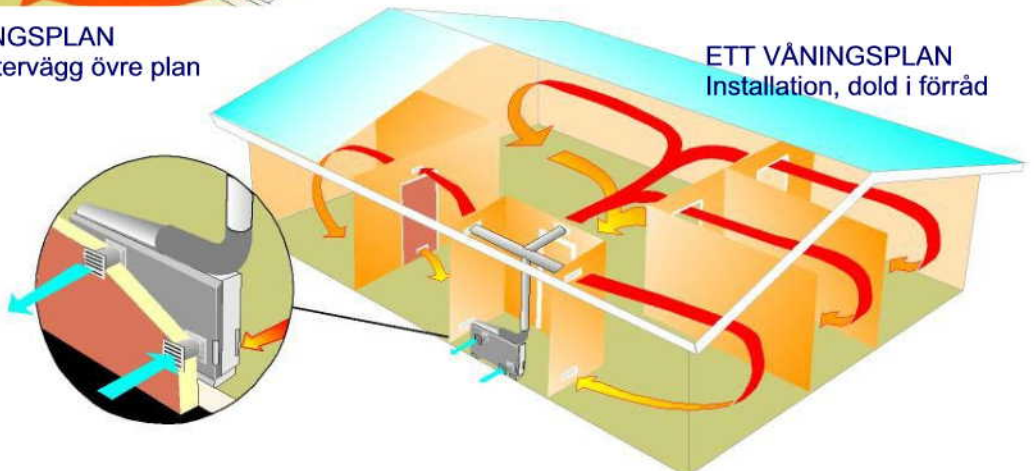
RECIRKULATION VIA TRAPPHUS
